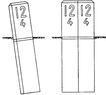
Fig. 76 Kilometermærke i beton fra BANERNES BYGNING OG Udstyrelse , DANSKE STATSBANER København, 1965 , side 91.
